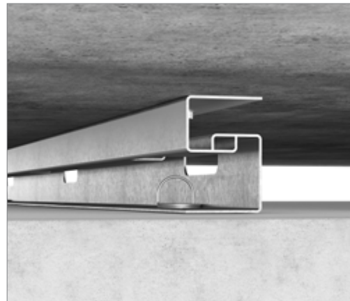
Direktbefestigungsschiene
